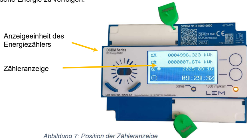
Abbildung 7: Position der Zähleranzeige
