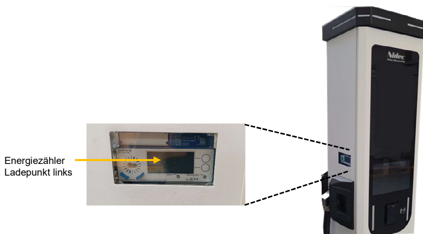
Abbildung 5: Position Energiezähler mit Public Key – linker Ladepunkt (LP1)
