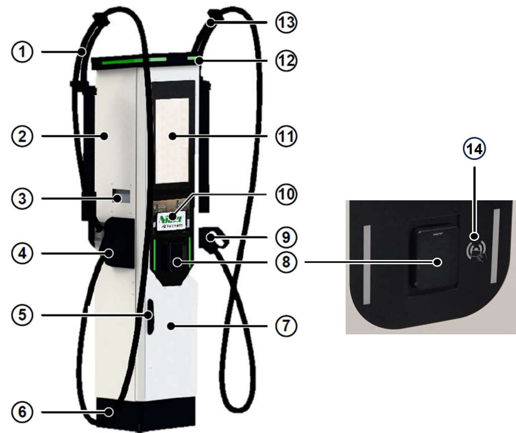
Abbildung 2: Außenansicht der Ladesäule
