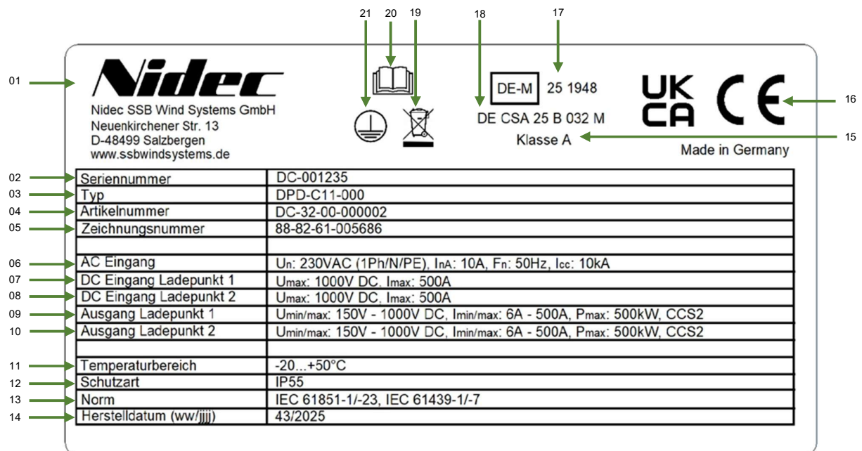
Abbildung 1: Typenschild
